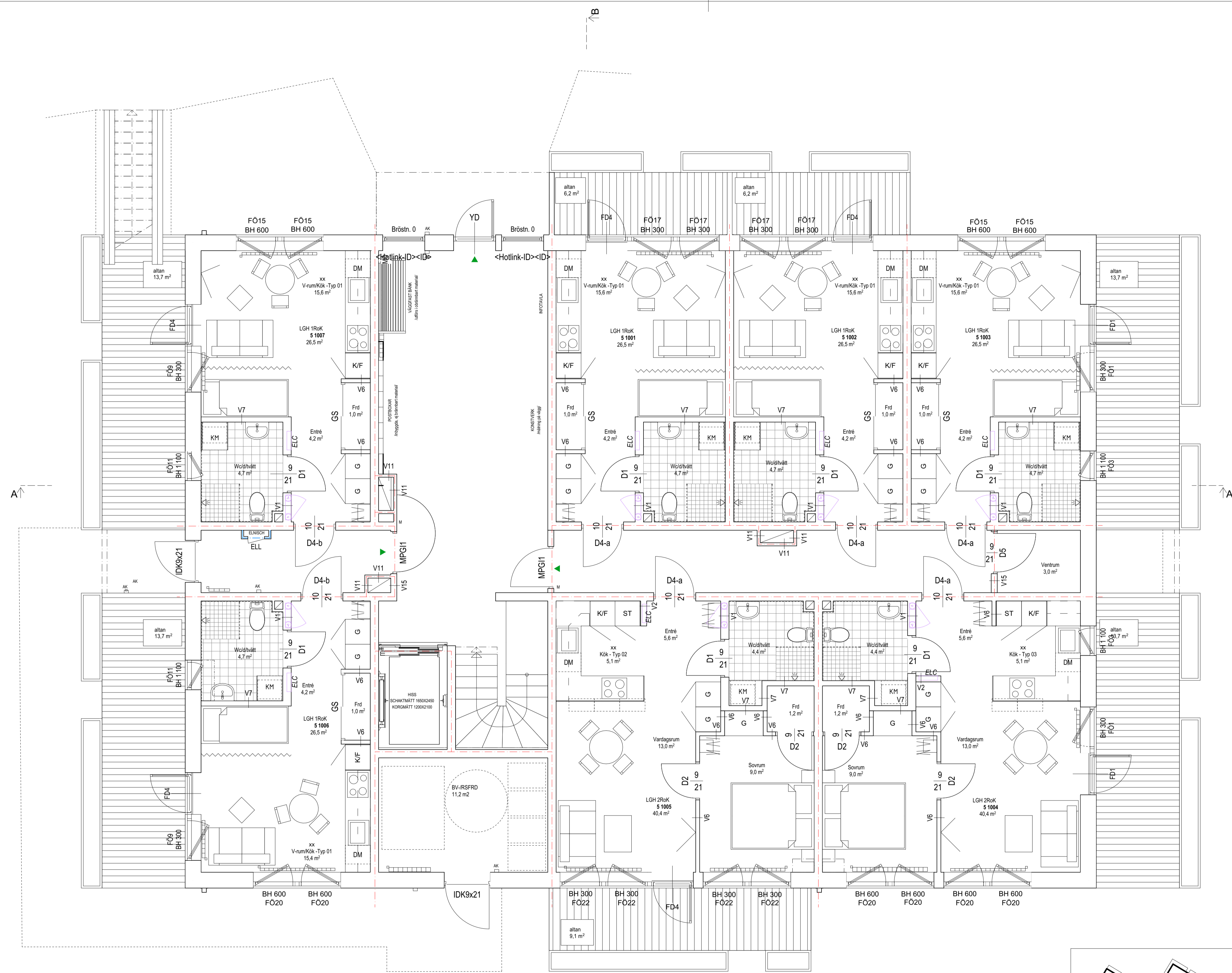
PLAN 10 1:50
