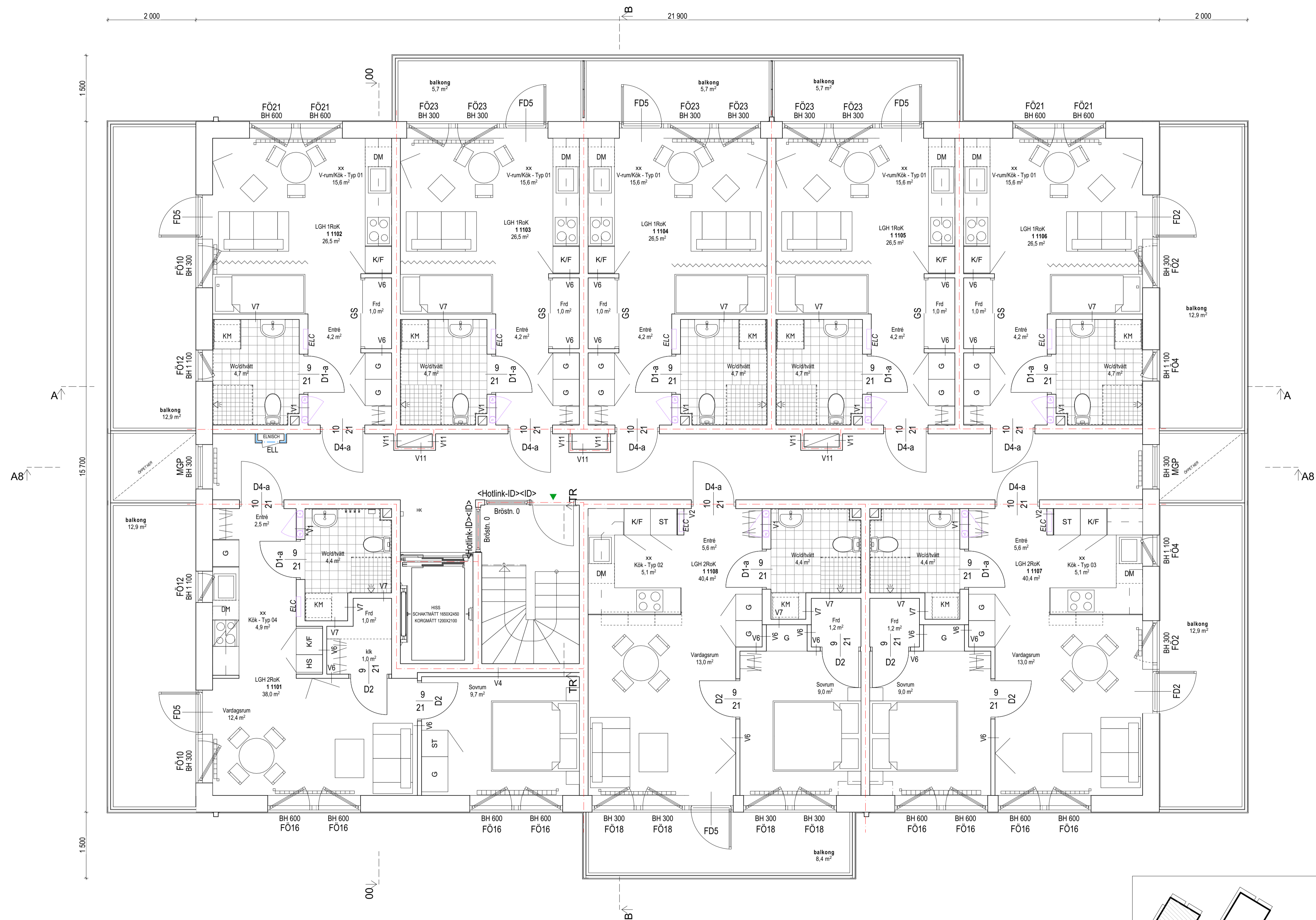
PLAN 11 1:50
