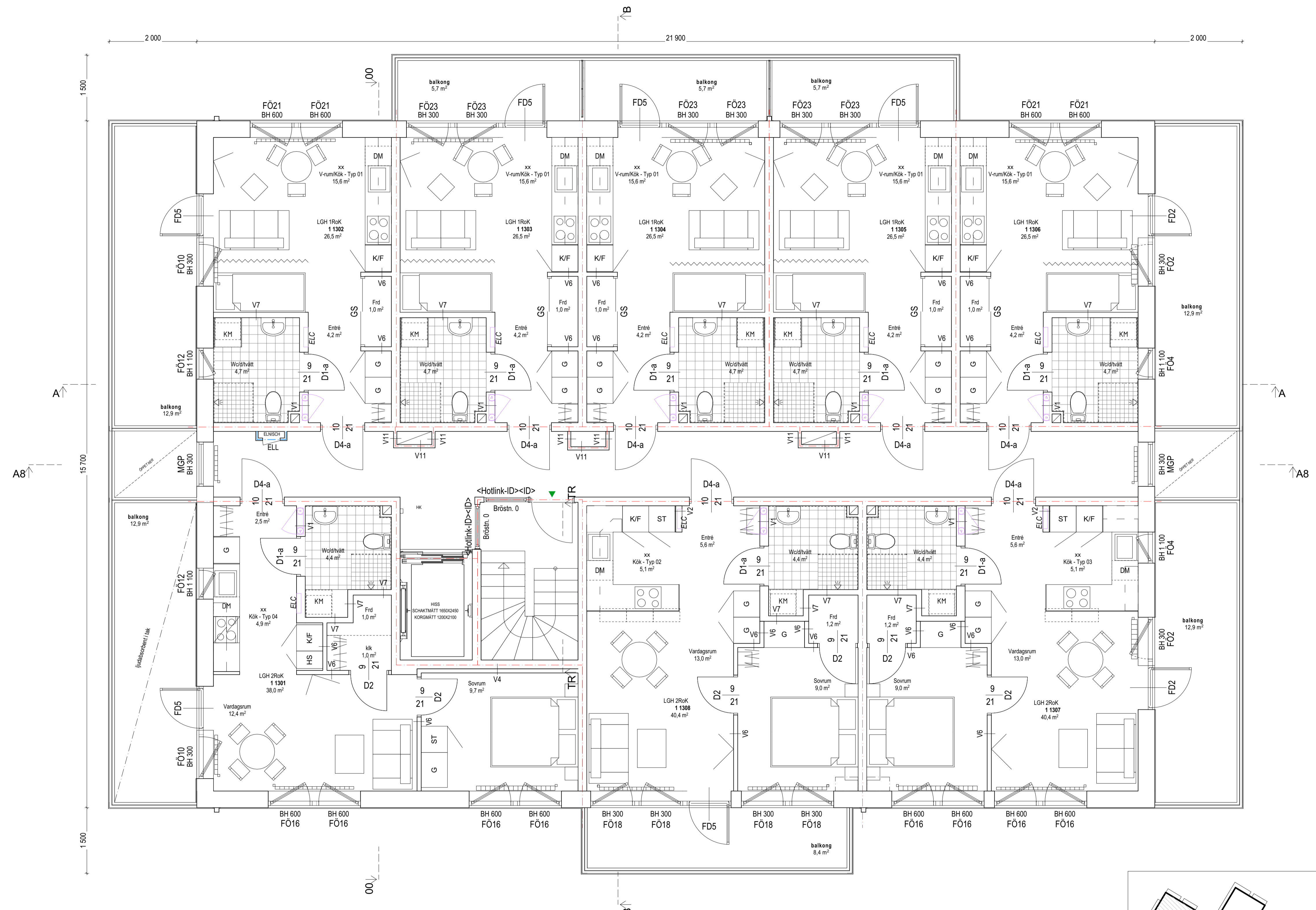
PLAN 13 1:50
