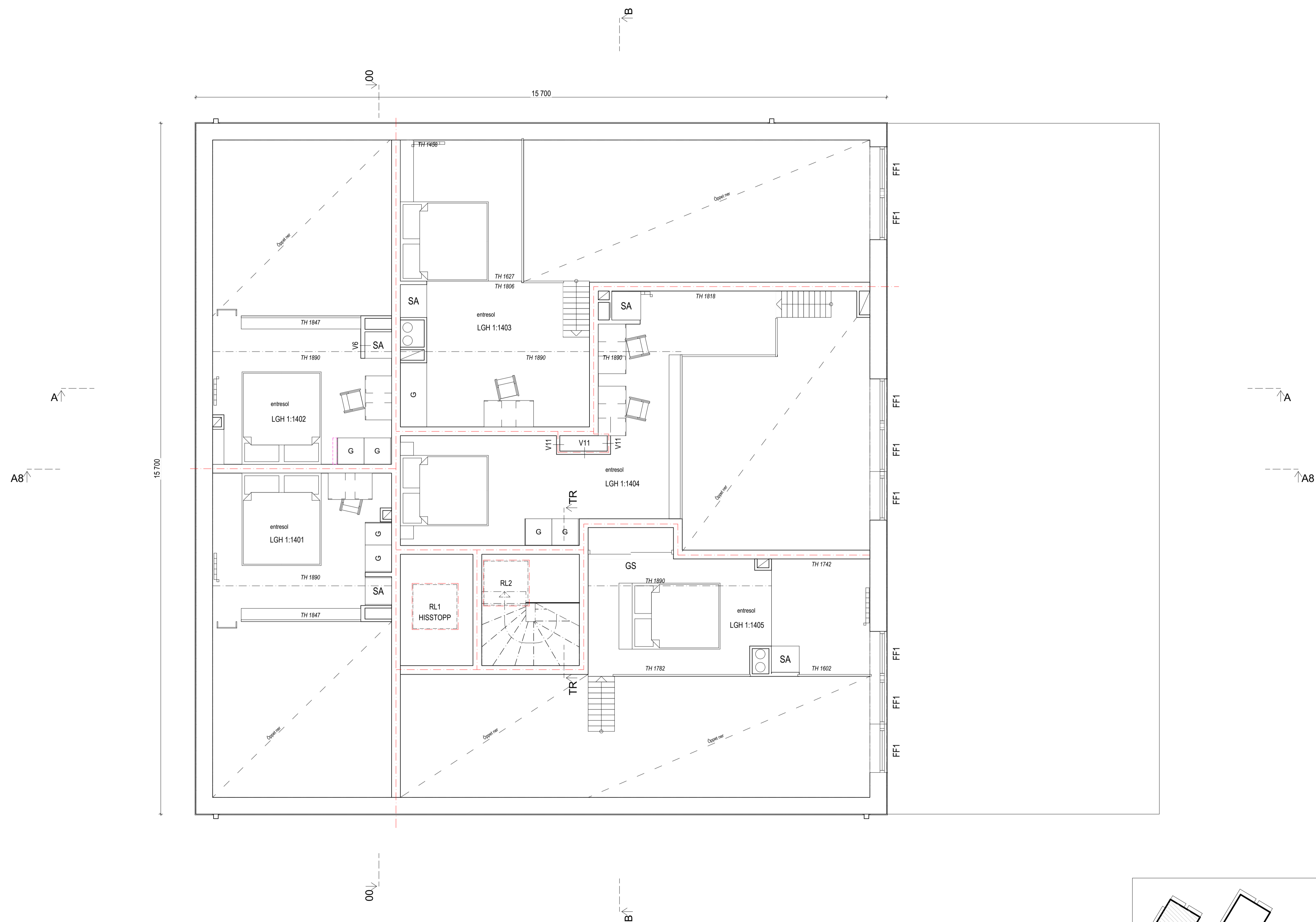
ENTRESOLPLAN 1:50
