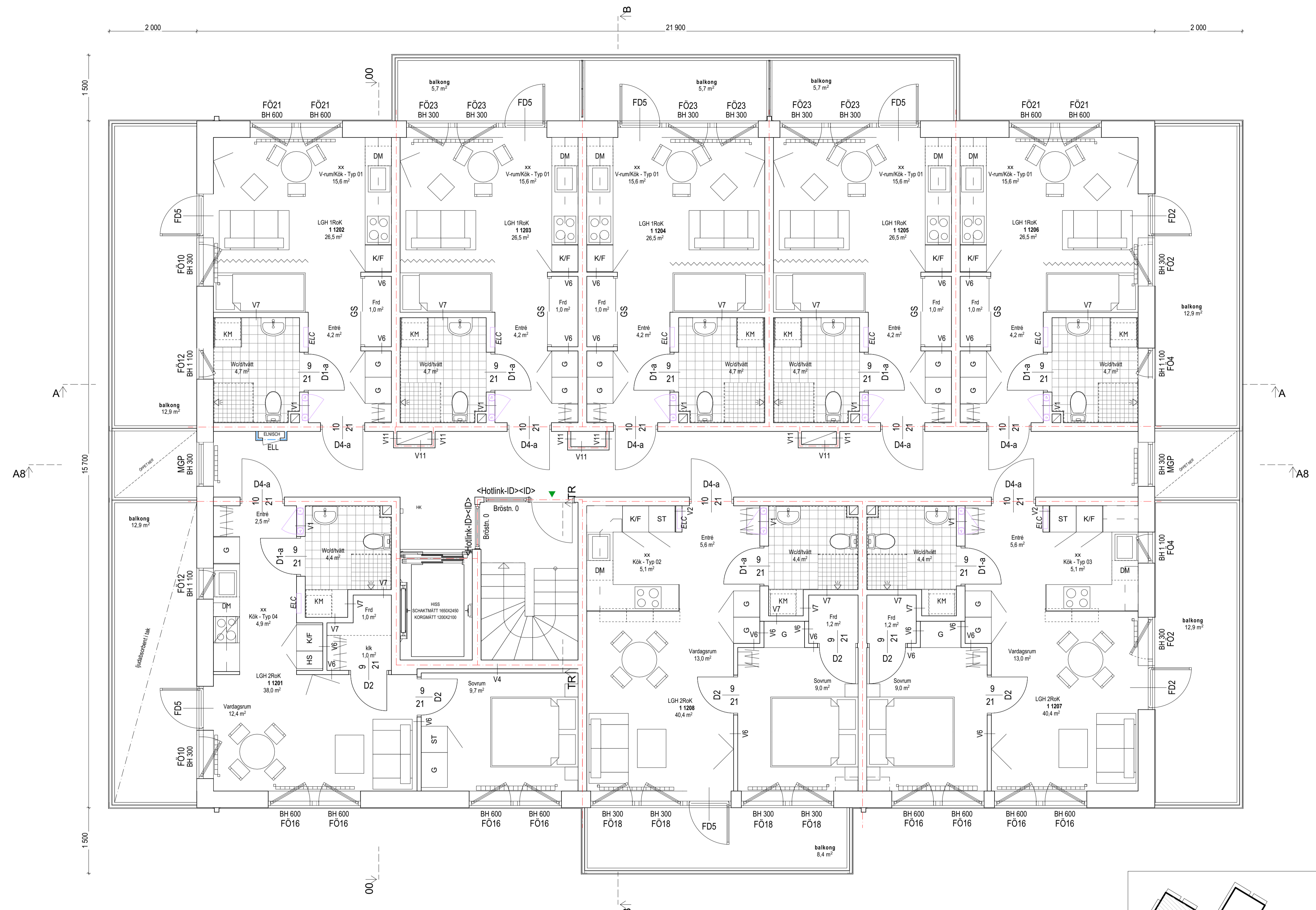
PLAN 12 1:50
